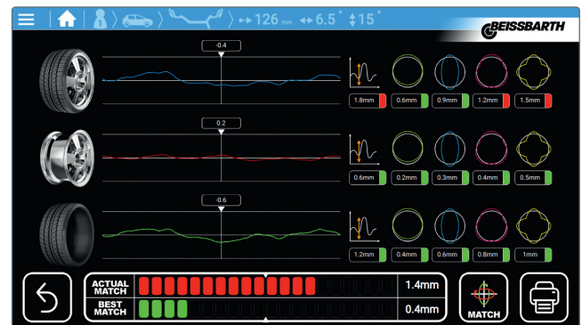
Eigenständiger Vorschlag der Match-Mount-Funktion
