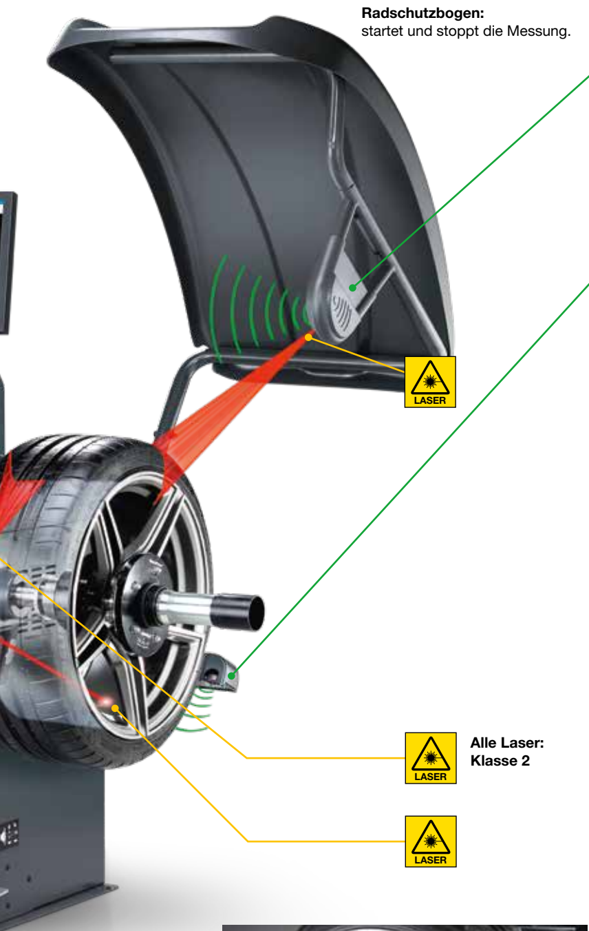
Zwei Sonare erfassen Speichenzahl, Raddaten, Zentrierung und Felgenschlag
