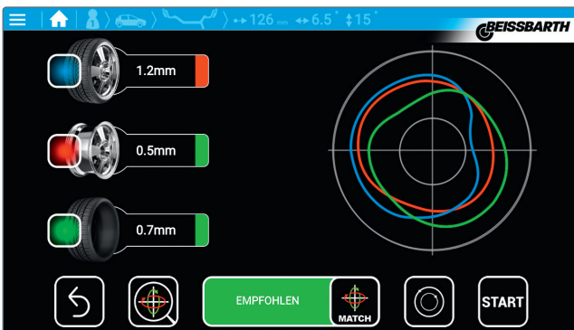
Schnelle Identifikation von Problemursachen
